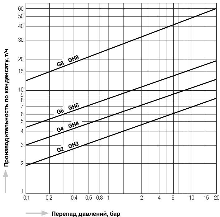
График производительности
